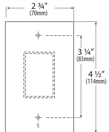
CM-30EE BOX
